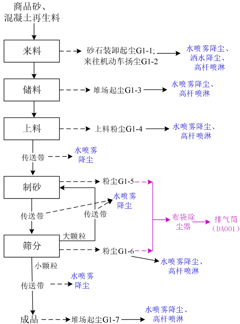
图 2-2 机制砂工艺流程及产污节点图
