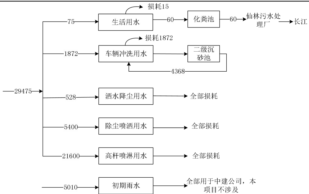
图 2-1 本项目年水平衡图 单位: t/a
