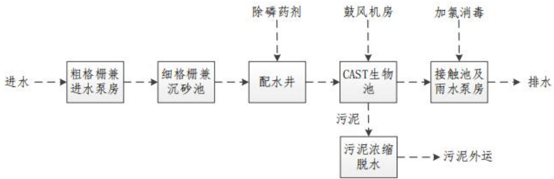
图4-2：仙林污水处理厂二期工艺流程图
